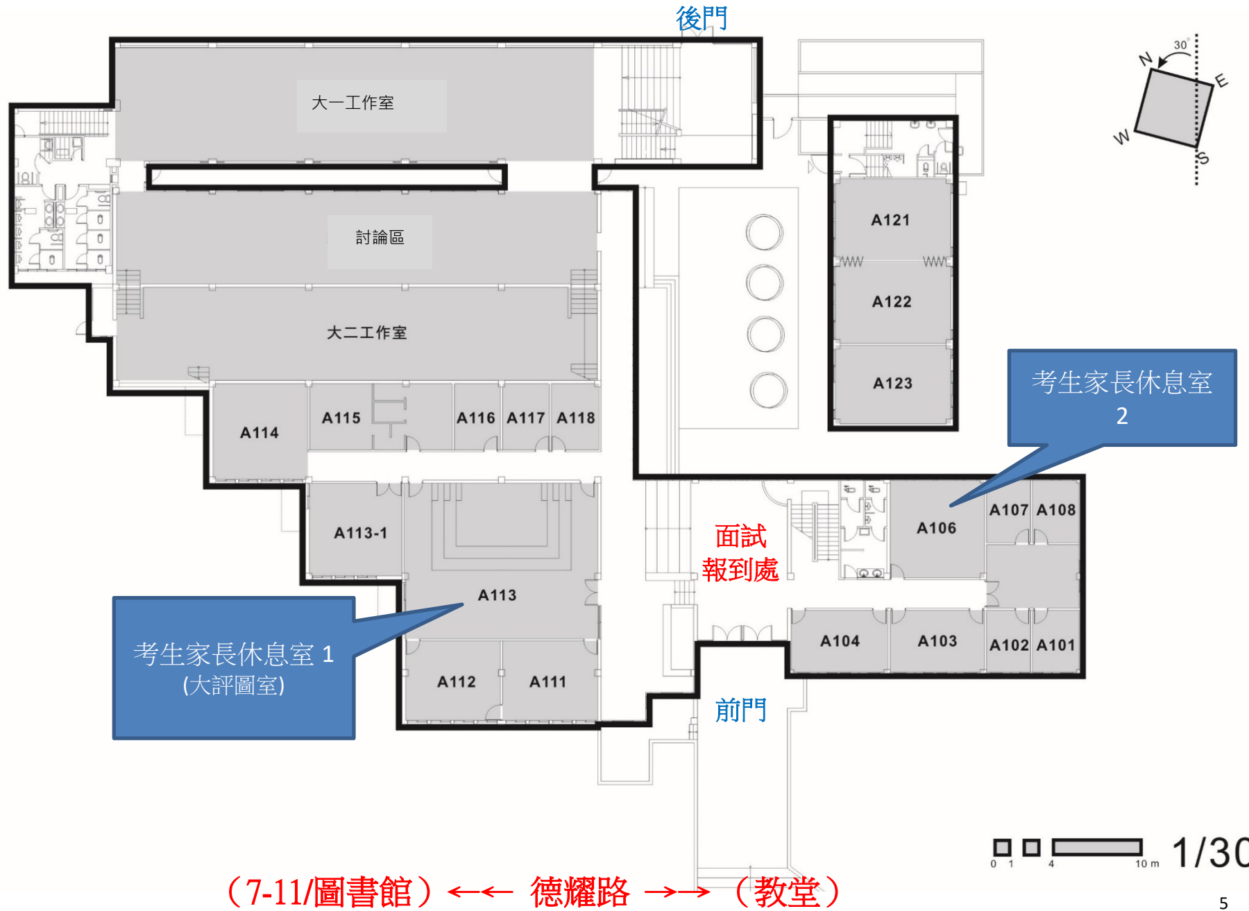
建築系館 1 樓平面圖
